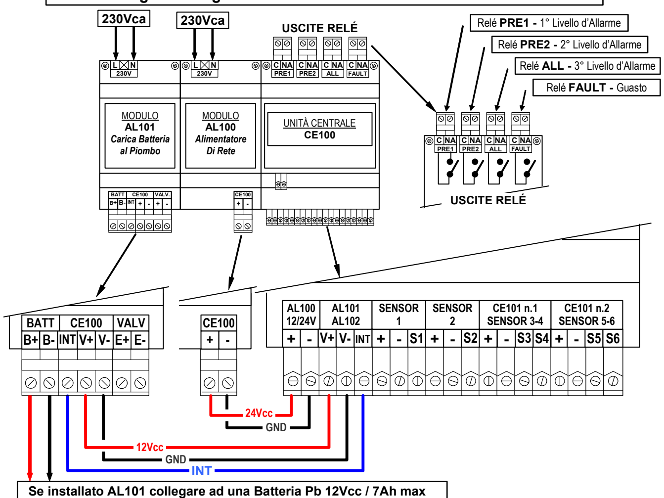
Fig 4– Collegamenti Alimentazione con il Modulo AL101
